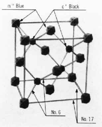
zincblende [H] [D] [M]
