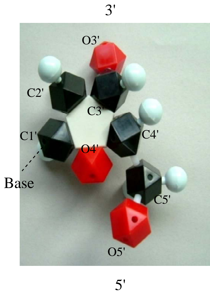
Deoxyribose
