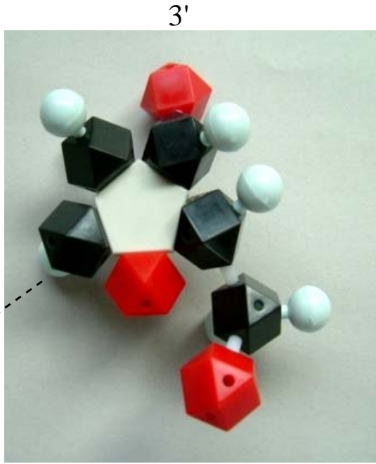
5' Deoxyribose
